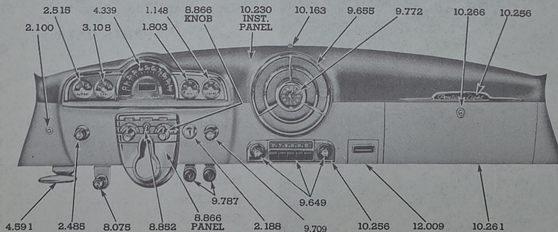
INSTRUMENT PANEL—1949 PONTIAC
