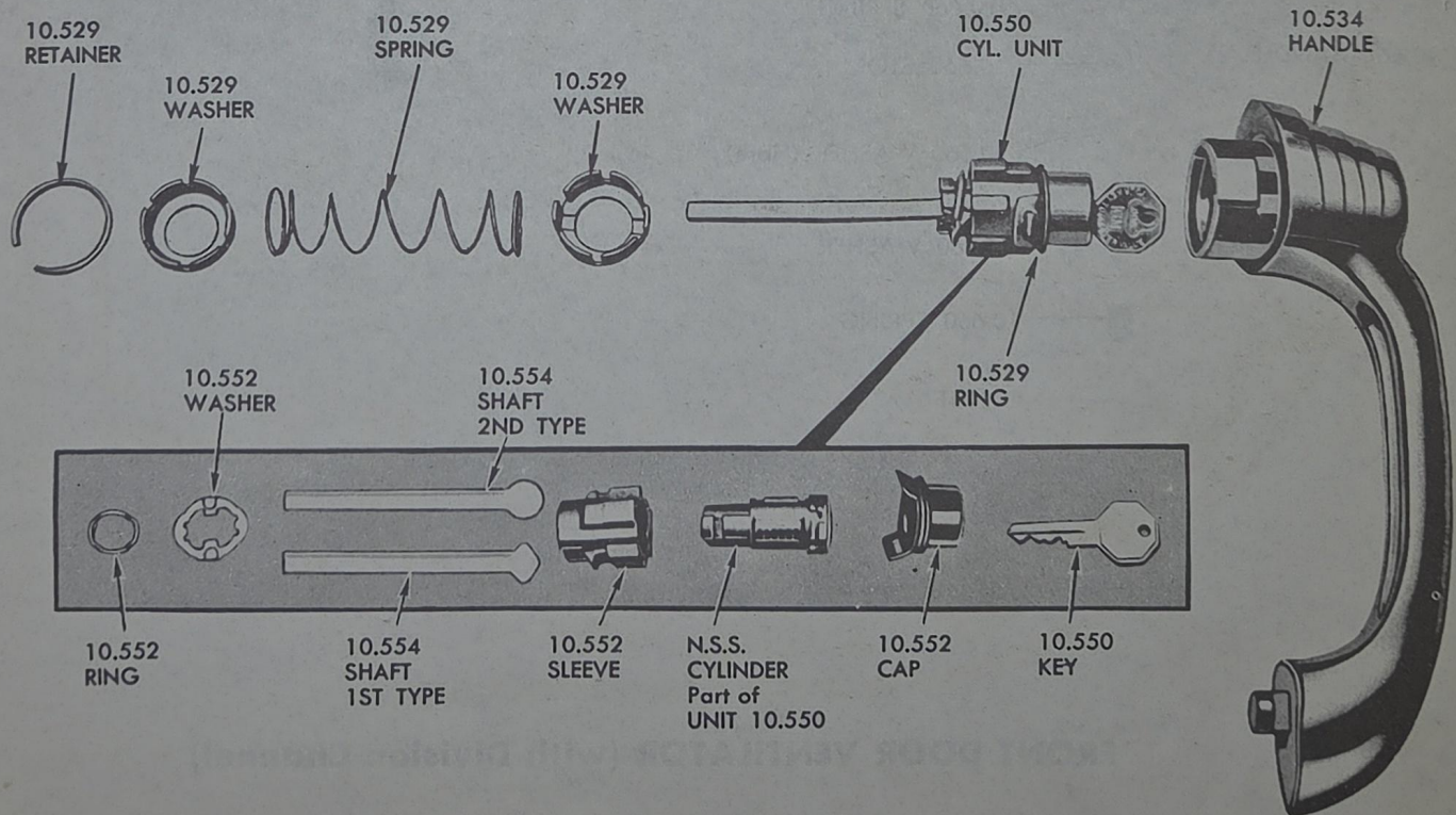
1949-51 DOOR LOCKING HANDLE
